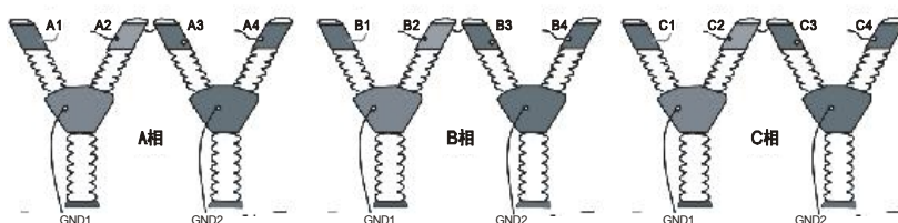
三断口信号线的连接
