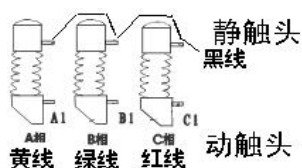
三断口信号线的连接
