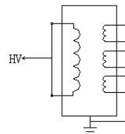
图 6-7 CT 接法
