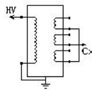
图 6-4 PT 末屏法
