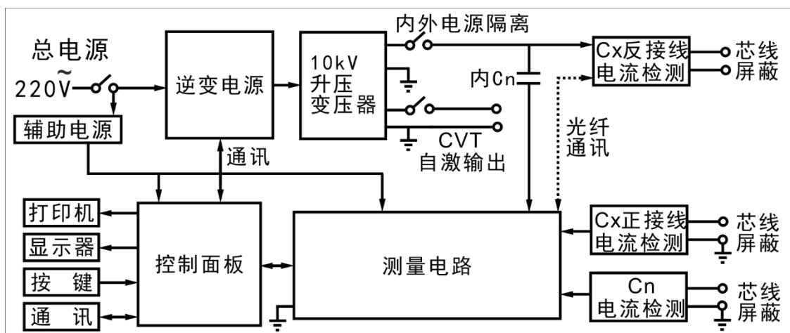
图 2—1 测量原理图
