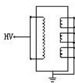
图 6-2 PT 接法
