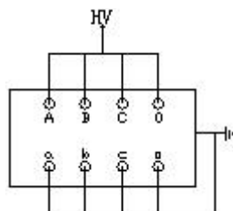
图 6-11 变压器反接法
