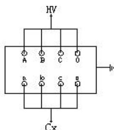
图 6-10 变压器正接法
