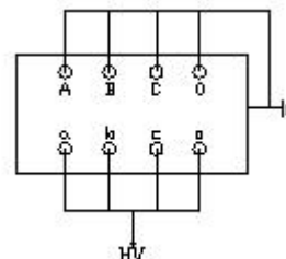
图 6-12 变压器反接法
