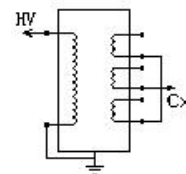
图 6-4 PT 末屏法
