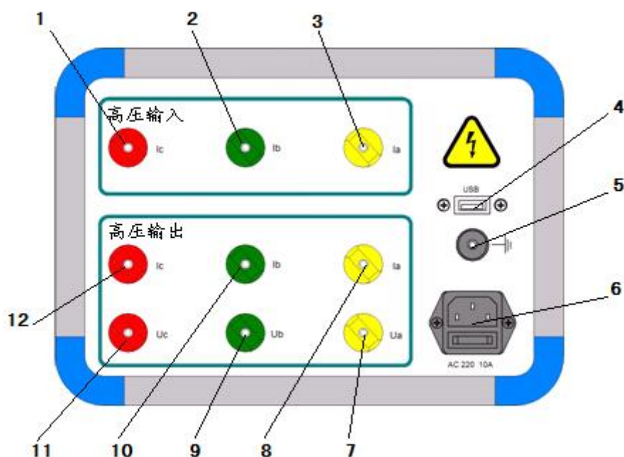
图 1b 变压器绕组变形综合测试仪背板图
