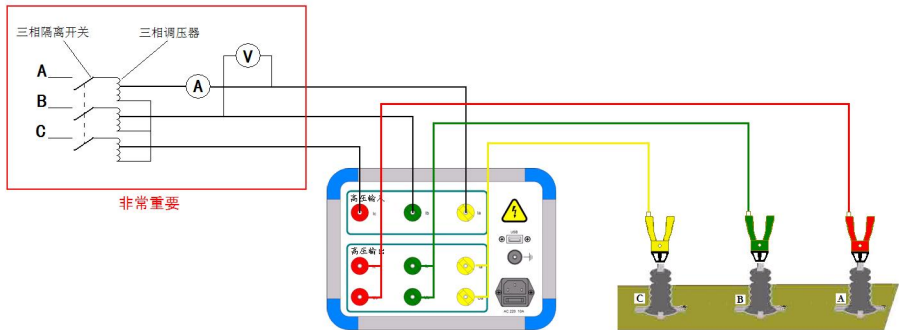
图 8 高电压短路阻抗法接线(后面板)
