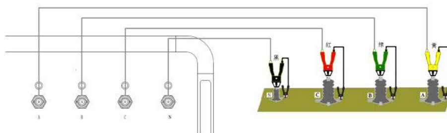
图 2 频响法测试接线图(三相自动测试)
