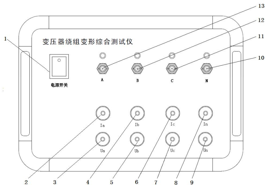
图 1a 变压器绕组变形综合测试仪面板图
