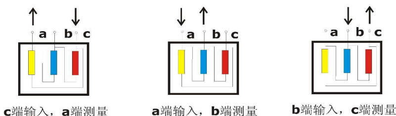
图 5 内连接△接线
