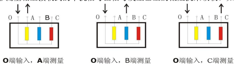
图 3 YN 接线
