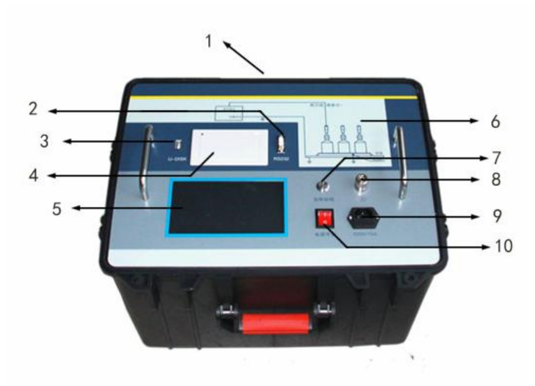
图三 面板示意图
