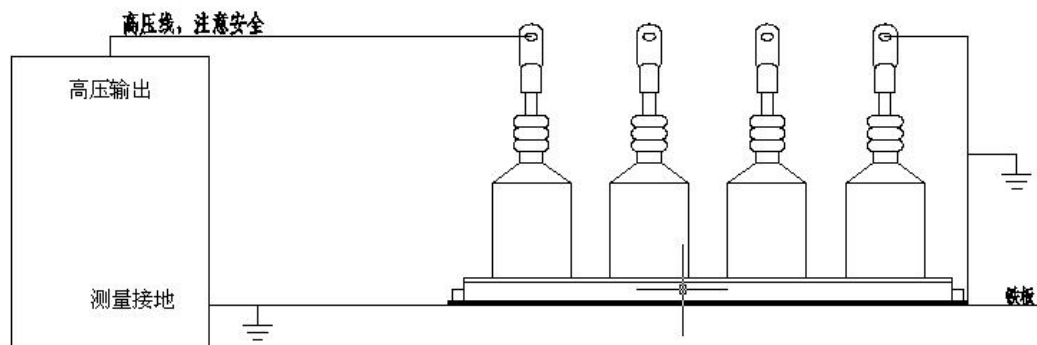
相地之间放电接线图(图二)
