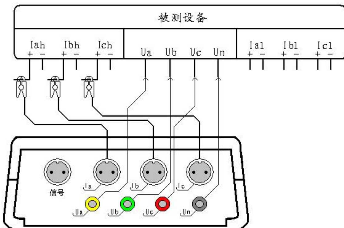
图十七、一次参量测试接线图
