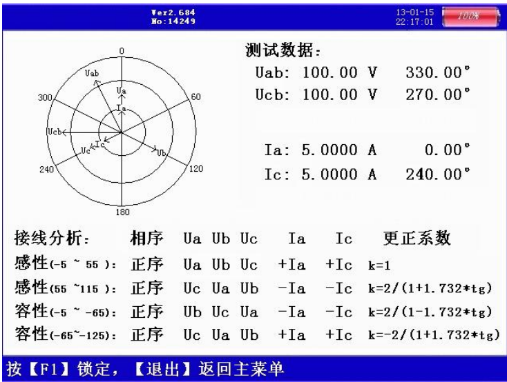
图九、三线计量
