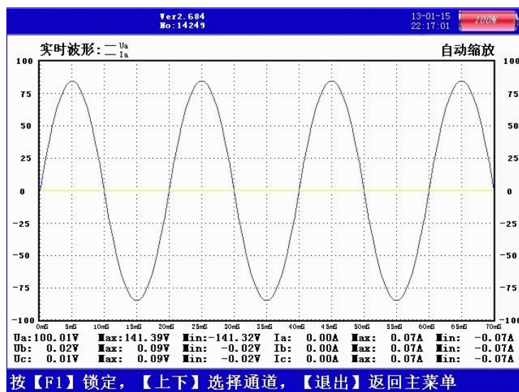
图十一、波形显示
