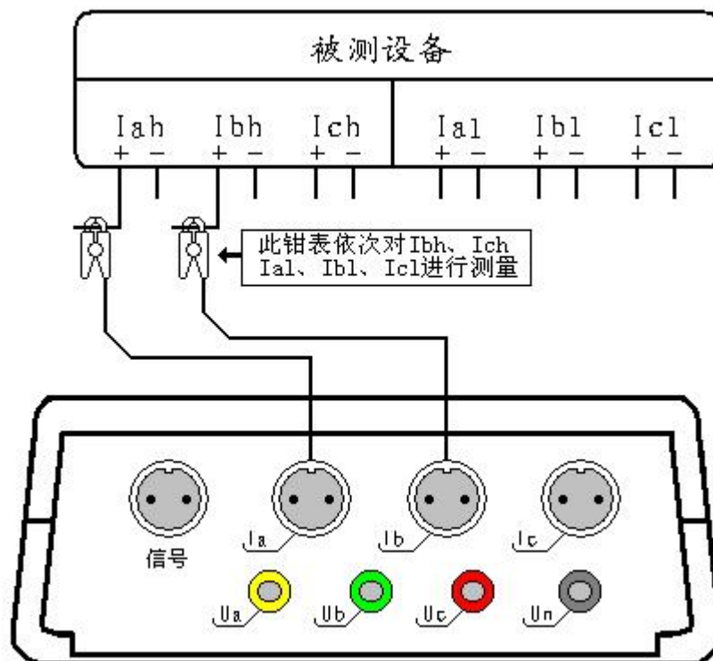
图十八、双钳差动接线图
