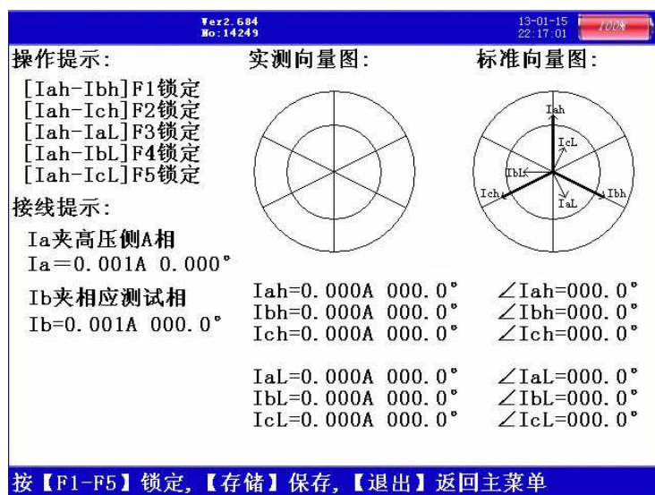
图八、双钳差动
