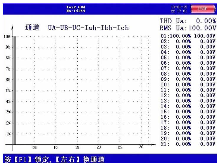
图十二、频谱分析
