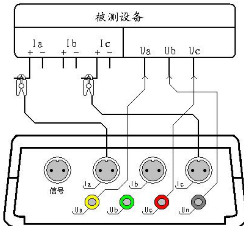
图十九、三线计量矢量测试接线图
