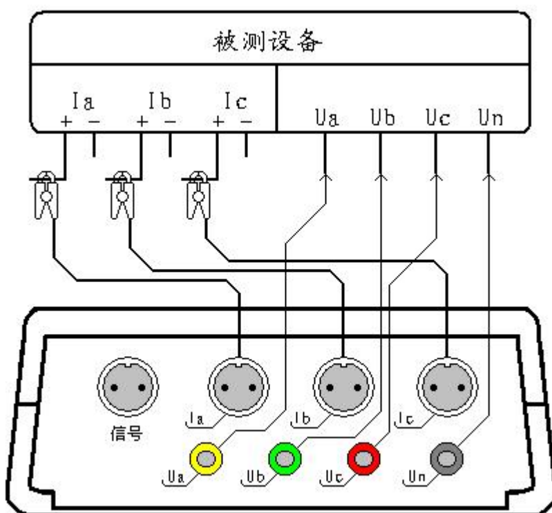
图十六、二次参量测试接线图
