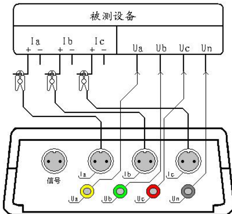
图二十二、谐波测试接线图
