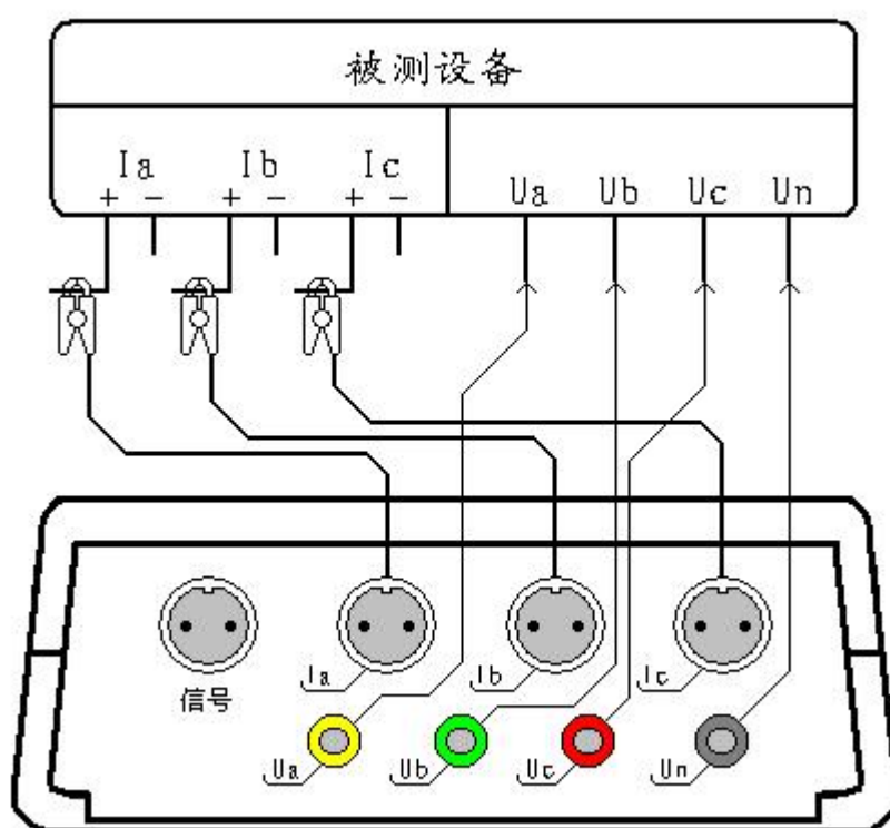
图十七、二次参量测试接线图
