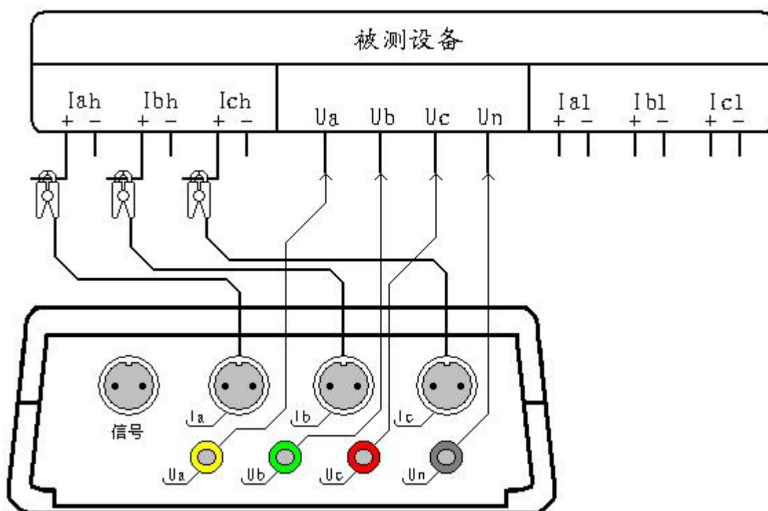
图十八、一次参量测试接线图
