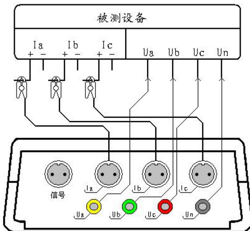
图二十一、波形显示接线图
