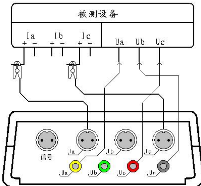
图二十、三线计量矢量测试接线图
