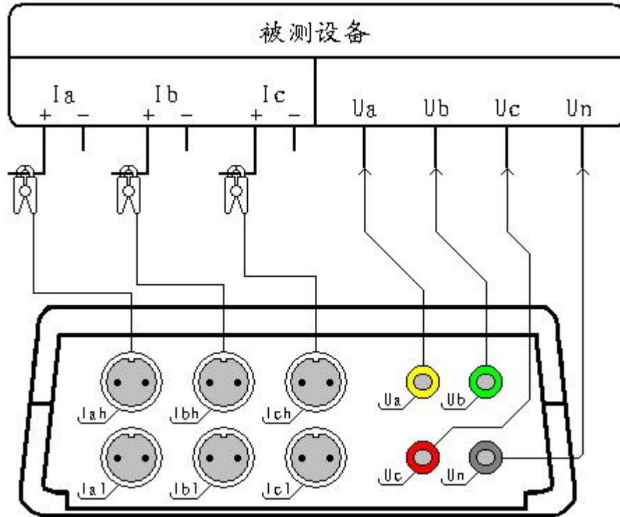
图二十五、谐波测试接线图
