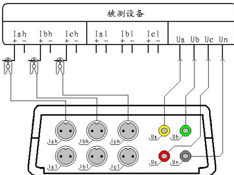
图十九、高压参量测试接线图
