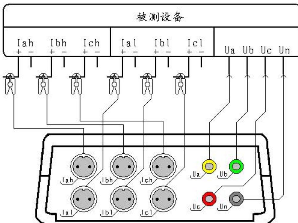
图二十三、波形显示接线图
