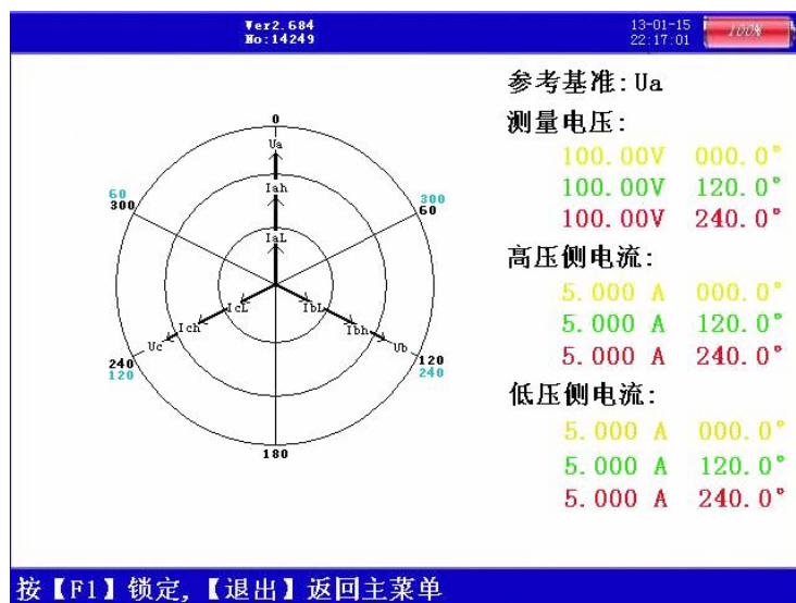
图六、二次参量
