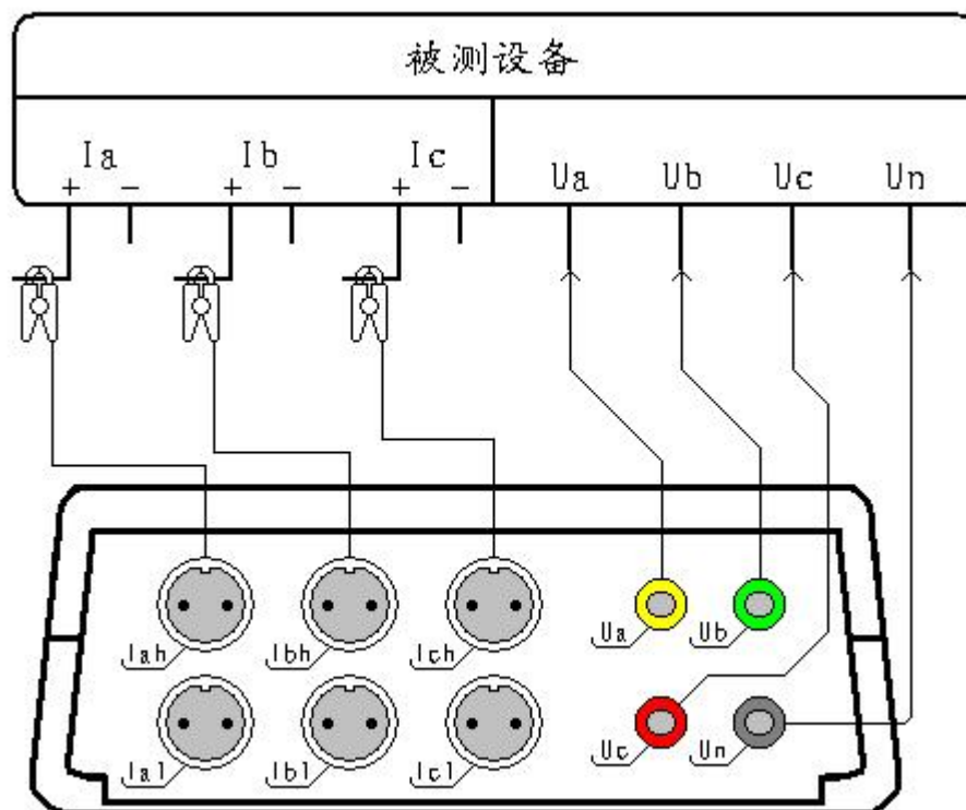
图二十五、谐波测试接线图
