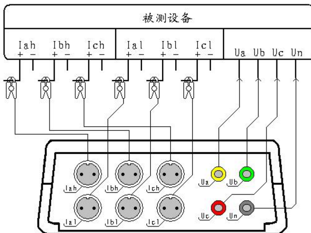
图十八、二次参量测试接线图
