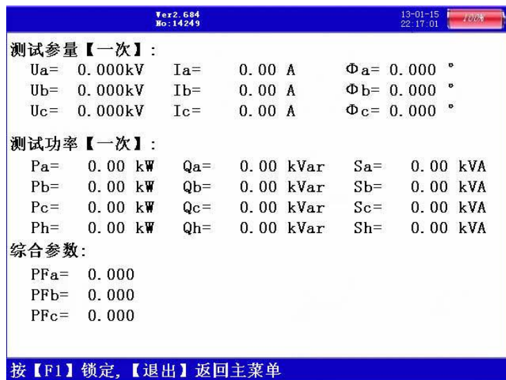
图七、一次参量
