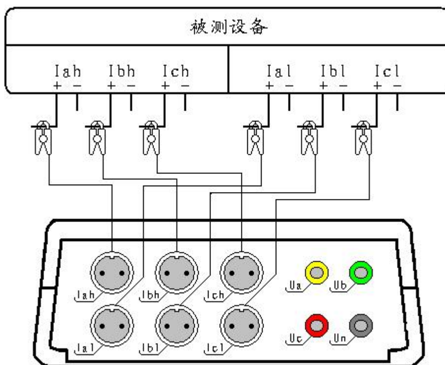
图二十、六钳差动接线
