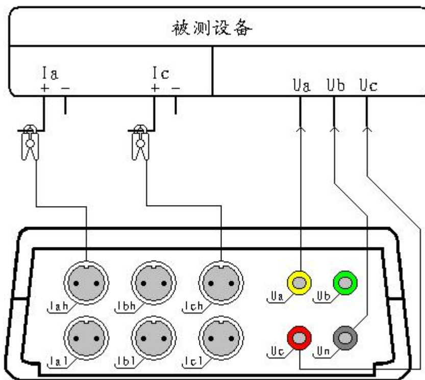
图二十二、三线计量矢量测试
