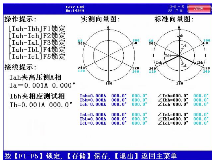
图九、双钳差动
