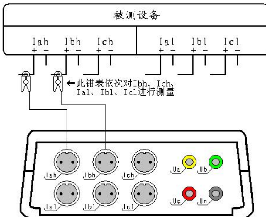
图二十一、双钳差动接线
