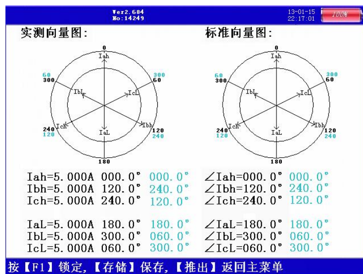
图八、六钳差动
