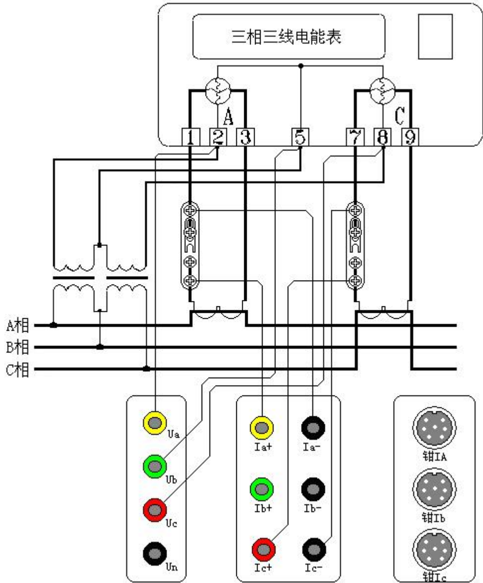
图二十四、三相三线高压计量表计直接接入测试
