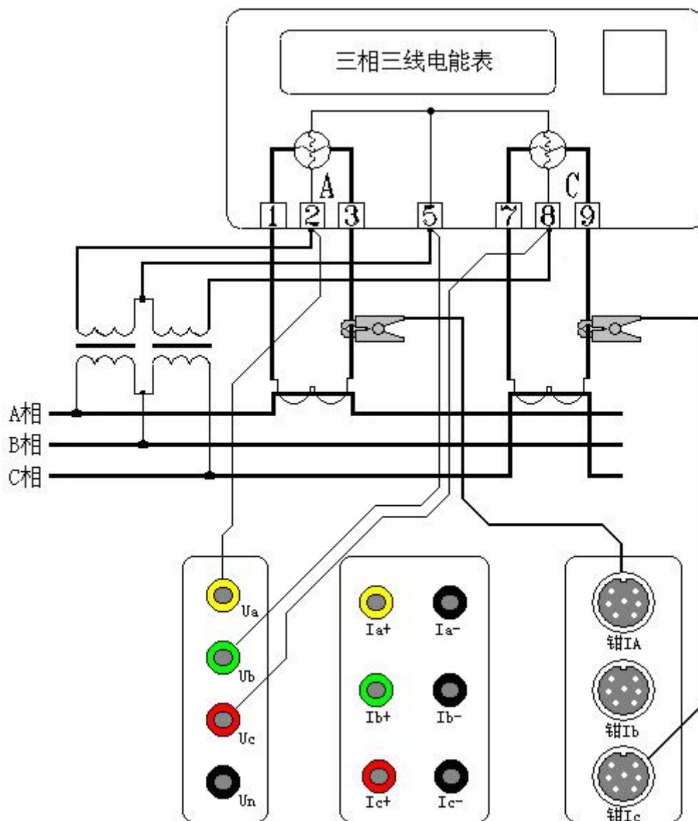
图二十三、三相三线高压计量表计经钳表接入测试
