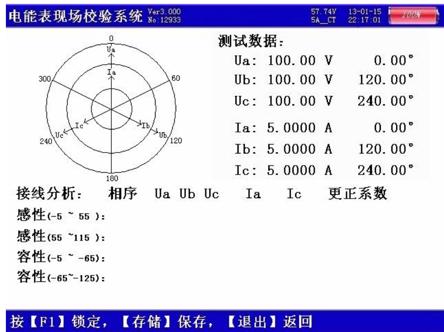
图八、矢量分析屏—三相四线
