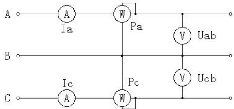
图十九、三相三线计量原理图
