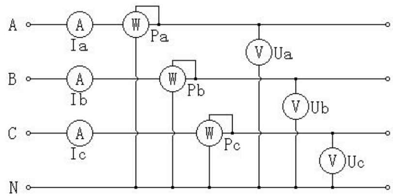
图二十、三相四线计量原理图
