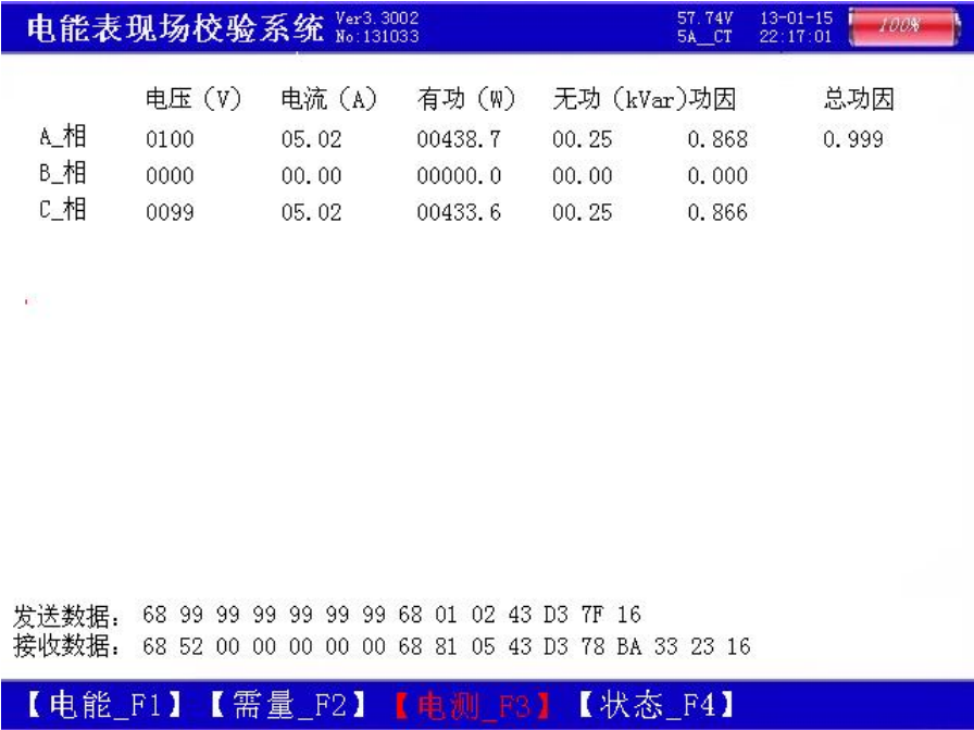
图十三、测试_485 电测 按 F4 显示现场表的工作状态如最近编程时间、需量清零时间、编程次数、需量清零次数、电池工作时间、电表日期、系统时间、最大需量周期、滑差时间、自动抄表日期等。
