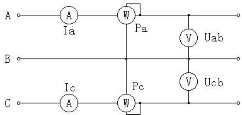
图二十一、三相三线计量原理图
