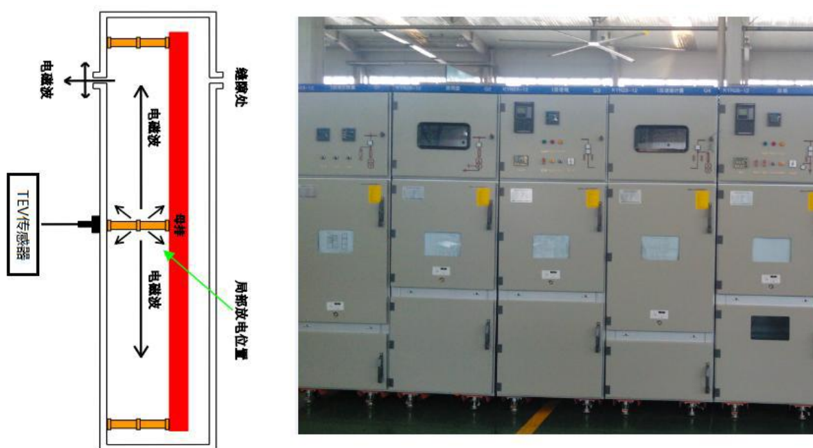
图 3-1 TEV 检测原理图
