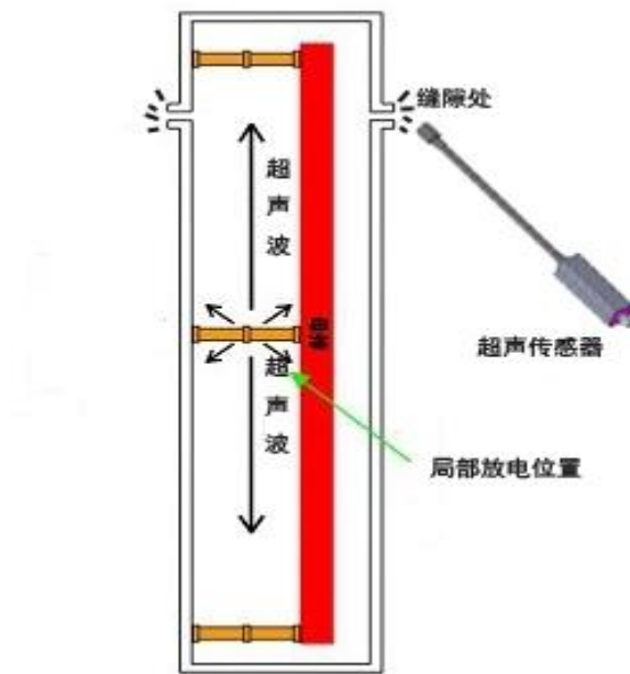
图 3-2 US 测量原理图
