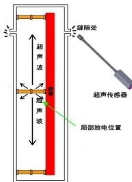
图 3-1 US 测量原理图
