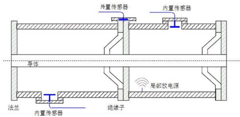
图 3-2 特高频测量原理图
