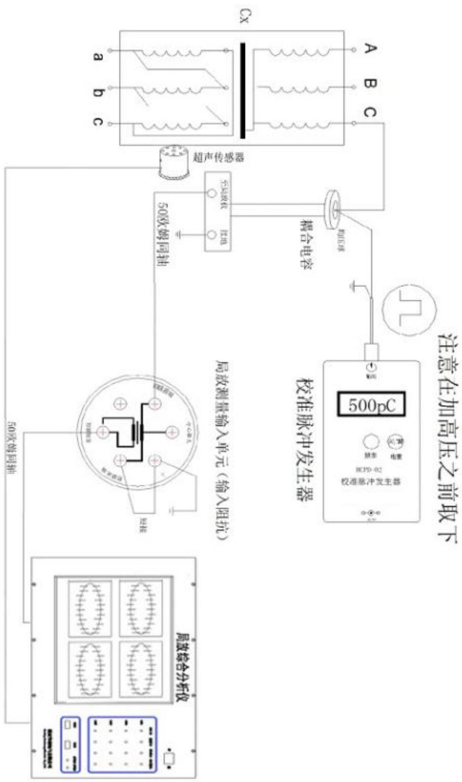
图 2 校准接线(外接耦合电容传输放电信号)
